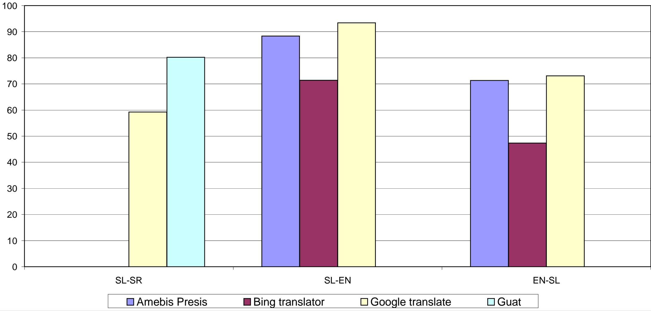
Vrednosti evalvacije z metriko WRR
